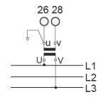
Voltage transf. Transf. Tensión
