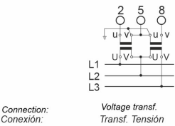
Esquemas de conexão Connections diagrams
