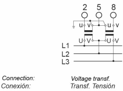
Esquemas de conexão Connections diagrams
