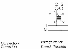
Esquemas de conexão Connections diagrams
