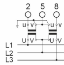
Connection: Conexión: Voltage transf. Transf. Tensión
