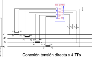
Conexión tensión directa y 4 TI's
