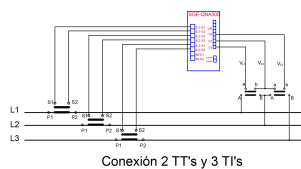
Conexión 2 TT's y 3 TI's
