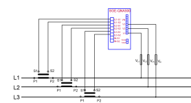
Conexión tensión directa 3 hilos y 3 TI's
