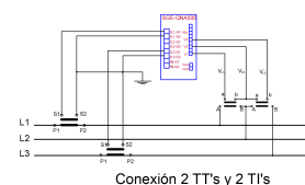
Conexión 2 TT's y 2 TI's
