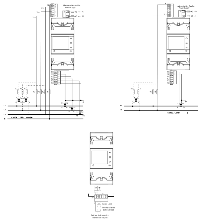
4W: 3Ph+N
