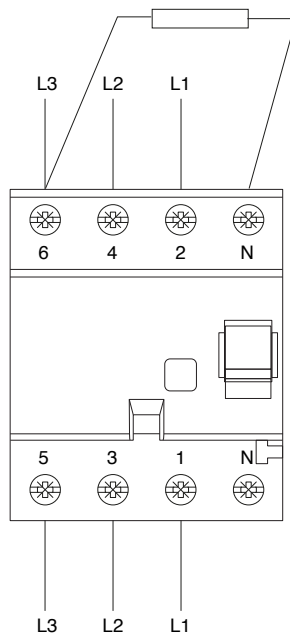
Connexion triphasée
