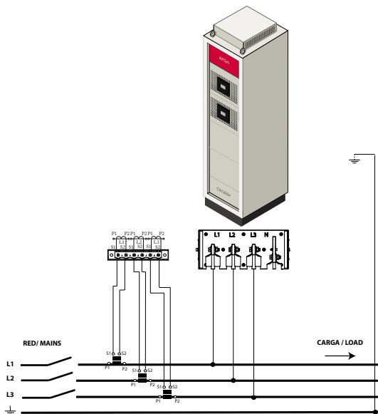
Medida trifásica con conexión a 3 hilos y medida de corriente en el lado de Red.
