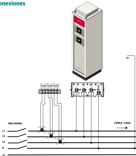
Medida trifásica con conexión a 4 hilos y medida de corriente en el lado de Red.
