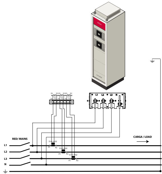
Medida trifásica con conexión a 4 hilos y medida de corriente en el lado de Carga.
